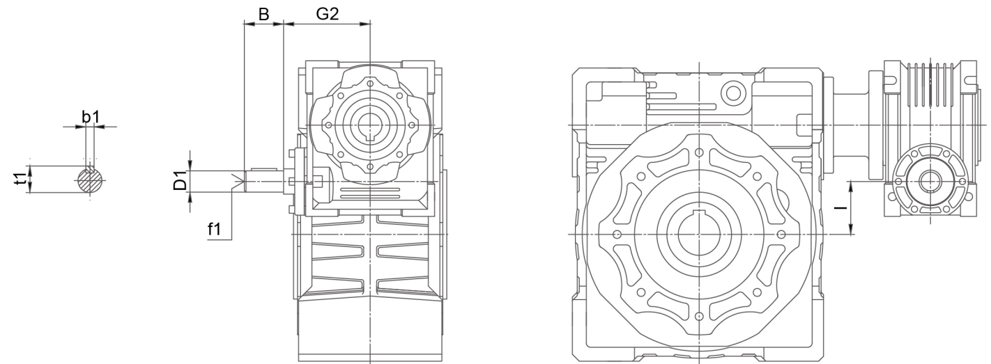
10.6 JRV+JMRV 尺寸图
