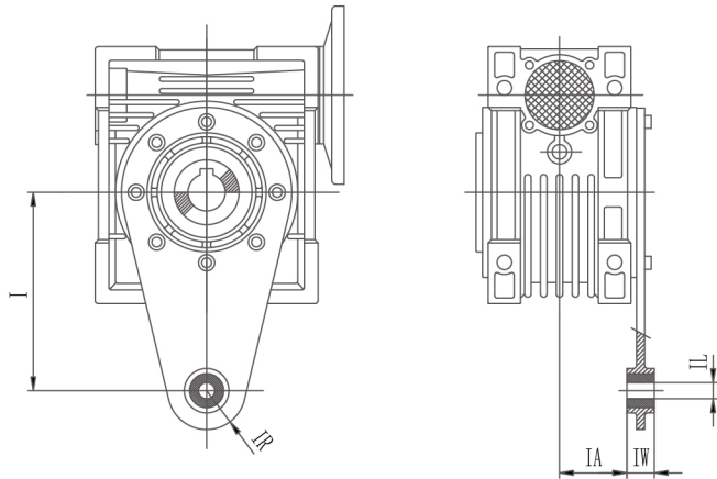
11.3 扭力臂
