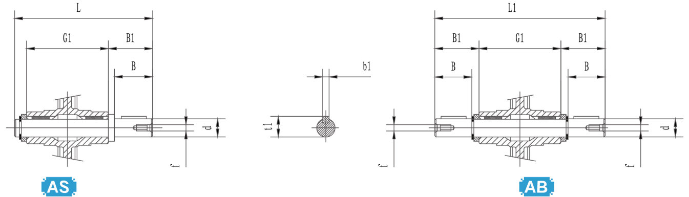
10.7 输出轴
