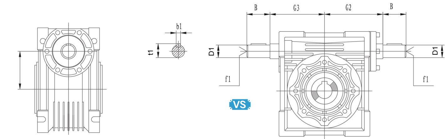
10.5 JRV 尺寸图
