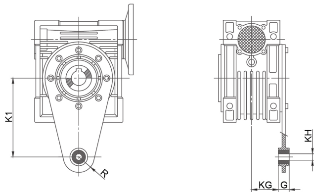
10.9 扭力臂
